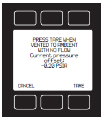
TARE PRESS
